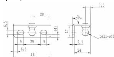
ST9699QU Ruostumaton kulmalaippa + kuula Ø10 mm, L=56, T=2,5
