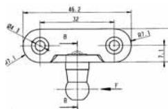
ST6284UG Vahvistettu kulmalaippa + kuula Ø10 mm. L=46, T=3
