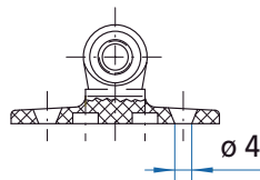
ST9584QE Kiinnike musta komp. silmutalle, L=49, T=4
