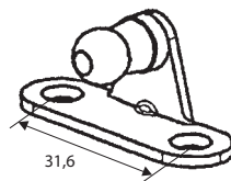
ST9222SJ Vahvistettu kulmalaippa + kuula Ø10 mm, L=46, T=3
