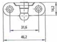
ST9222SJ Vahvistettu kulmalaippa + kuula Ø10 mm, L=46, T=3
