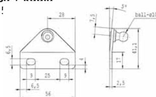
ST9699QU Ruostumaton kulmalaippa + kuula Ø10 mm, L=56, T=2,5
