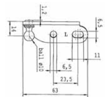
ST1361NN Kulmarauta 101°A vasen + kuula Ø10 mm
